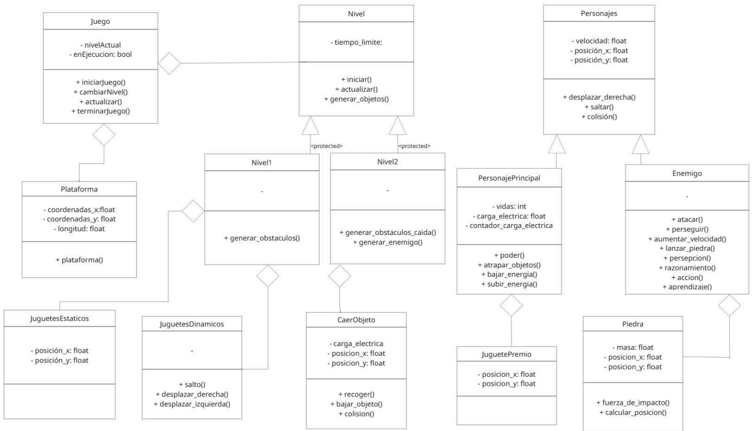
Diagrama 2. Diagrama de clases, proyecto final
