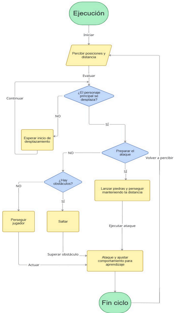
Diagrama 1. Diagrama de flujo de agente inteligente
